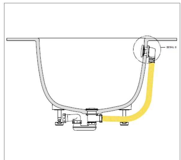
Seitenschnitt
