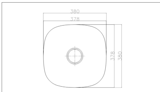
Grundriss
