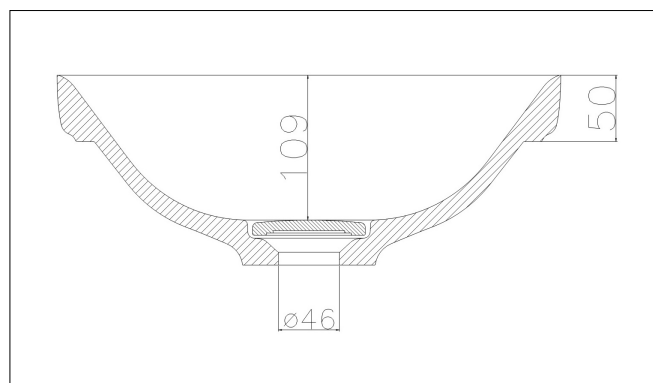
Ansicht
