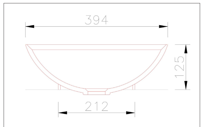
Seitenschnitt
