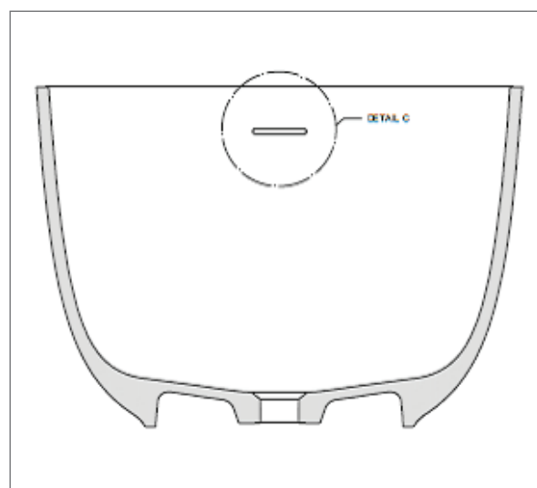
Seitenschnitt
