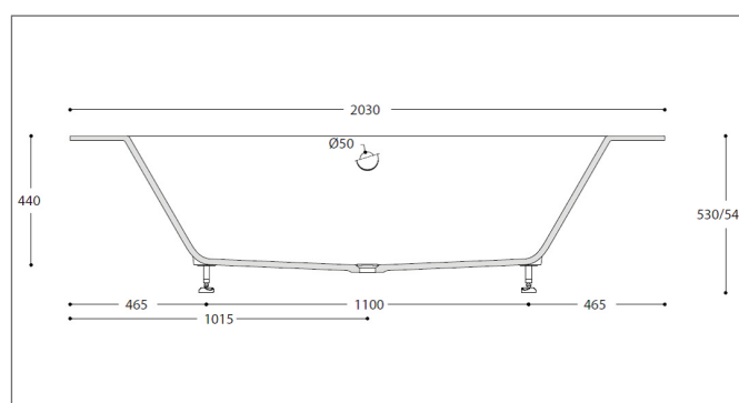
Ansicht
